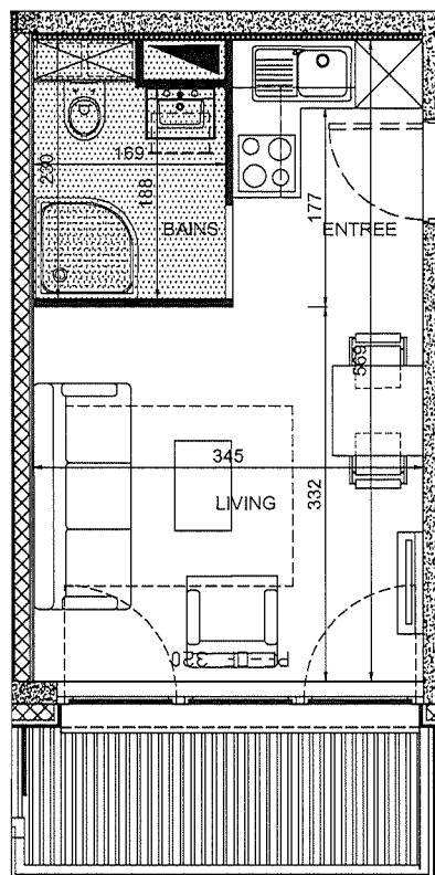
PLAN DE L'APPARTEMENT 8.08
