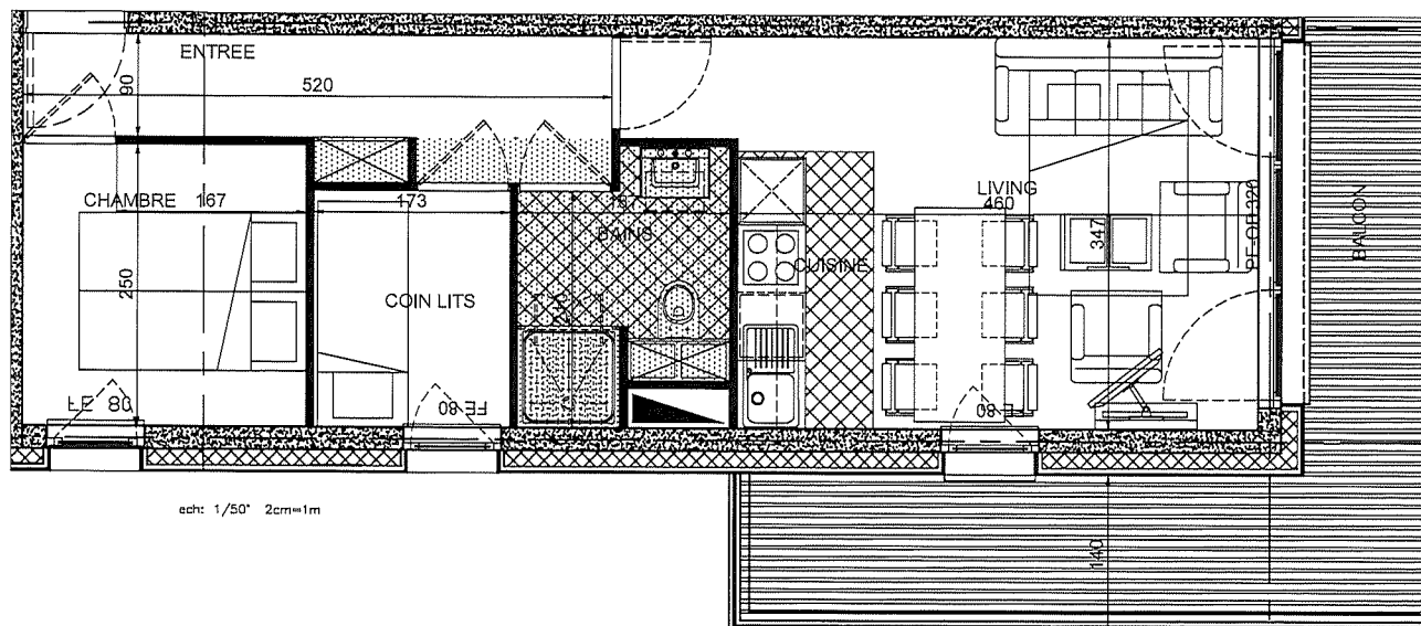
PLAN DE L'APPARTEMENT 4.07
