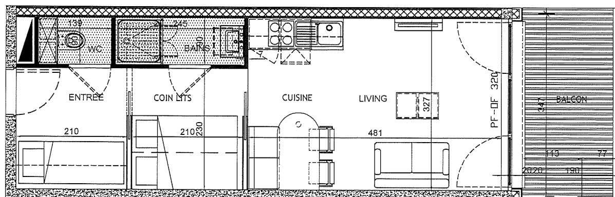
PLAN DE L'APPARTEMENT 4.05
