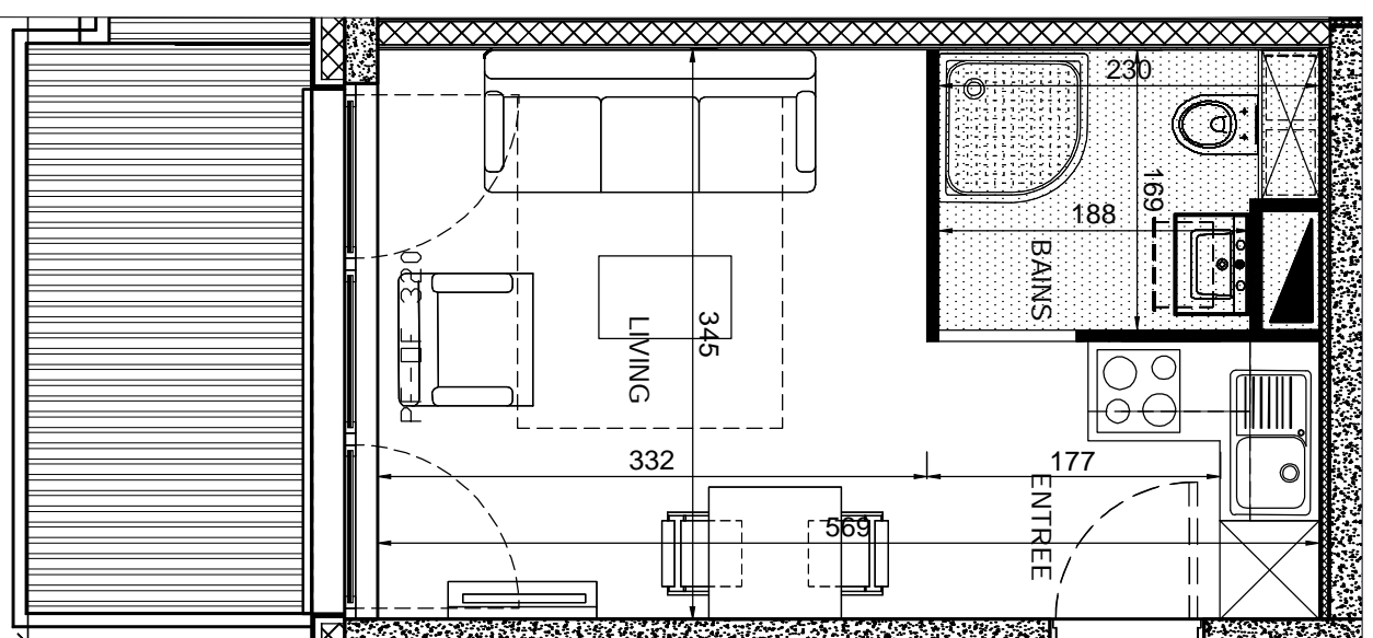
PLAN DE L'APPARTEMENT 5.08
