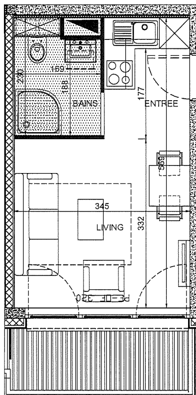
PLAN DE L'APPARTEMENT 6.08
